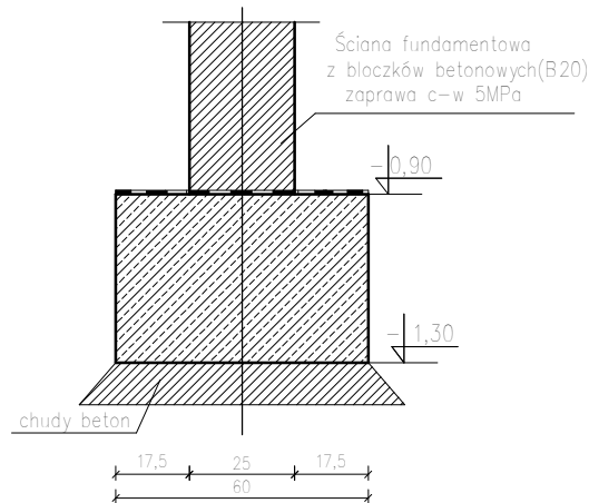
Ława fundamentowa Ł1 skala 1:20
