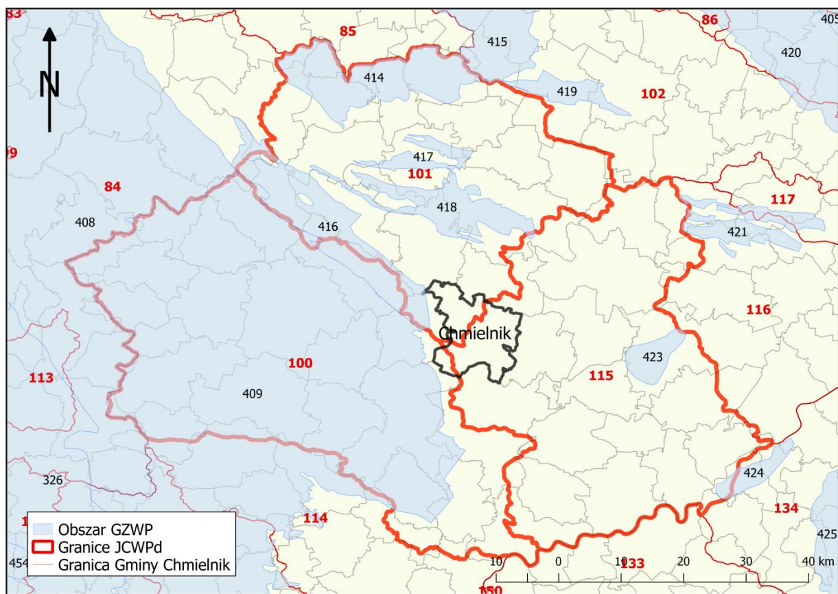
Map. 8 Położenie Gminy Chmielnik na tle obszarów GZWP i JCWPd
