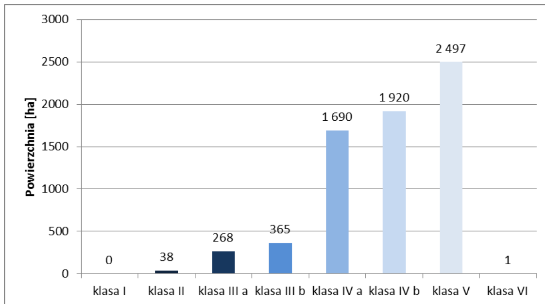
Wyk. 5 Klasyfikacja gruntów ze względu na klasę w Gminie Chmielnik
